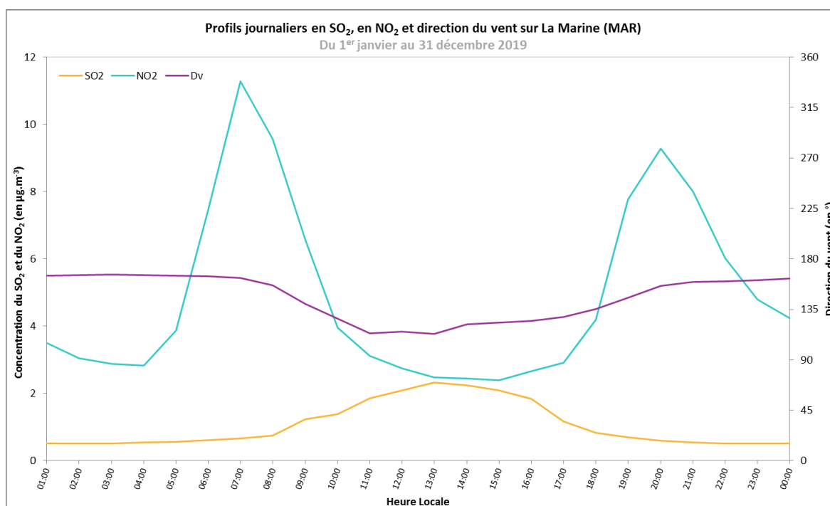
Figure 5 : Evolution des profils journaliers de SO 2 (µg/m 3 ) et de NO 2 (µg/m 3 ) ainsi que celle de la direction du vent (°) sur la station MAR du 01/01/2019 au 31/12/2019.
