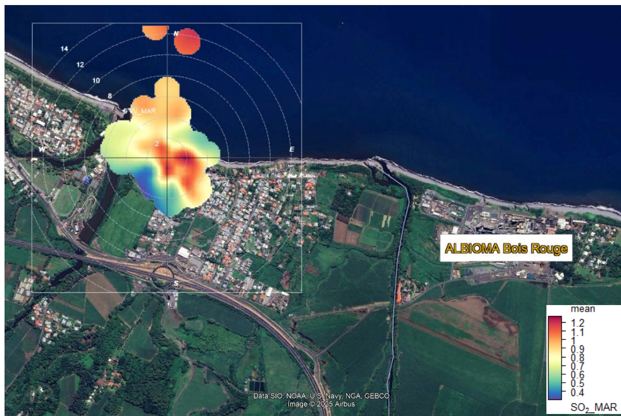
Figure 6 : Roses de pollution en \text{SO}_2 sur la station MAR au cours de l'année 2024.
