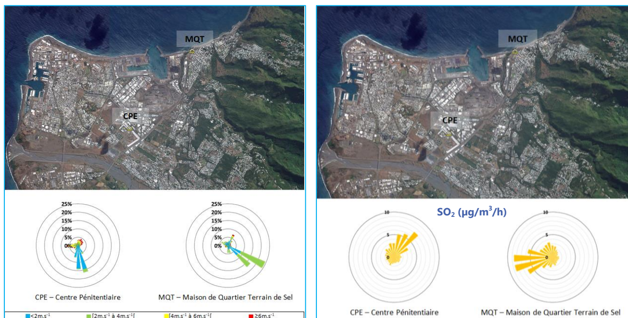
Figure 6 : Roses de vent et de pollution du SO 2 (µg/m 3 /h) sur MQT et CPE du 1 er janvier 2018 au 31 décembre 2018.
