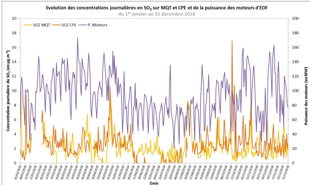
Figure 4 : Evolution des concentrations journalières en SO 2 sur les zones MQT et CPE ainsi que celles de la puissance des moteurs de la centrale EDF du 1 er janvier 2018 au 31 décembre 2018.
