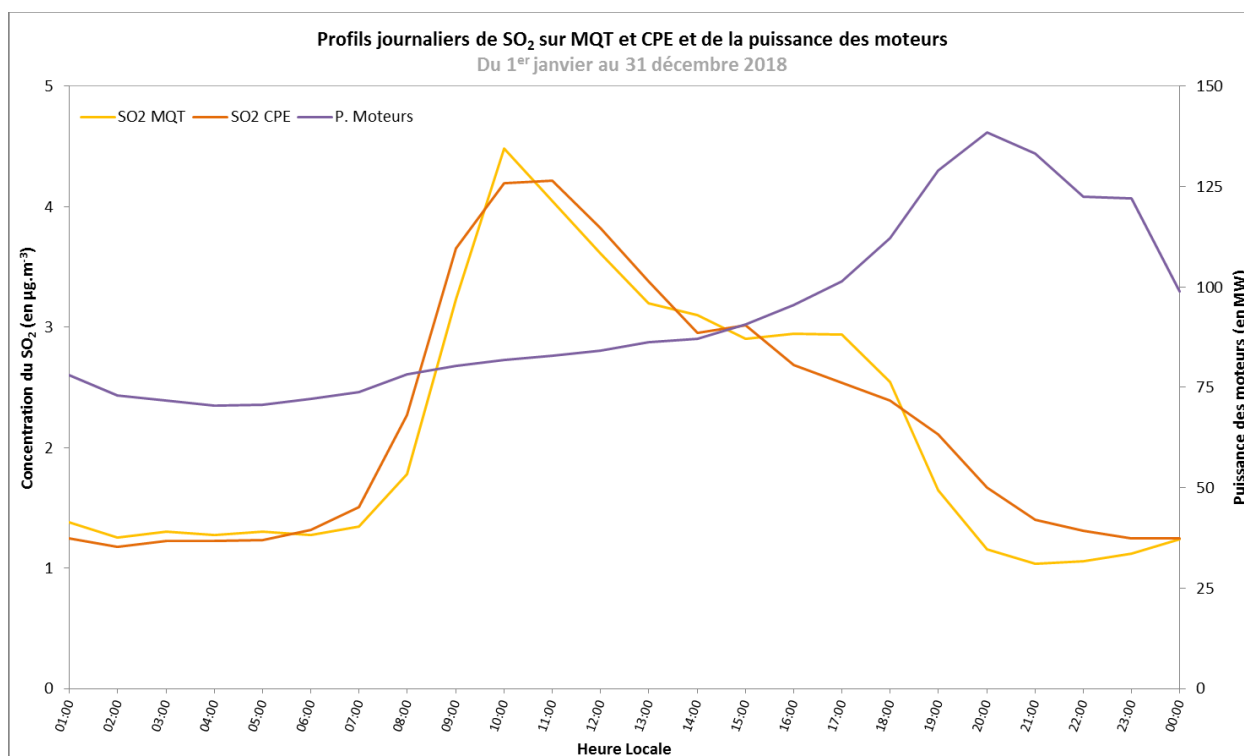
Figure 5 : Evolution des concentrations horaires moyennes en SO 2 (µg/m 3 ) sur les zones MQT et CPE ainsi que celles de la puissance moyenne des moteurs d'EDF du 01/01/2018 au 31/12/2018.
